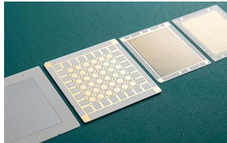
電子部品用回路基板（厚膜印刷基板）
